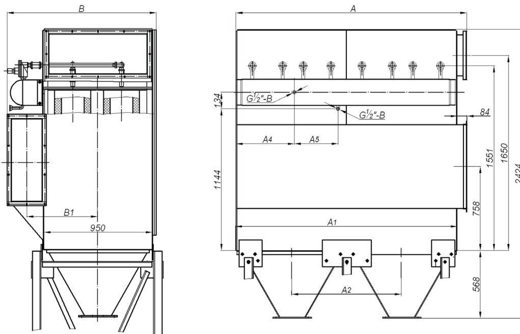
Рис. 7 Схема фильтра ФПИ-6; ФПИ-8
