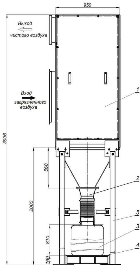
Рис. 1 Схема фильтра ФПИ-4 со стандартными опорами 1- фильтр ФПИ; 2- переходник ПЕМК; 3 - емкость для пыли (100 л); 4 - поддон; 5 - опора
