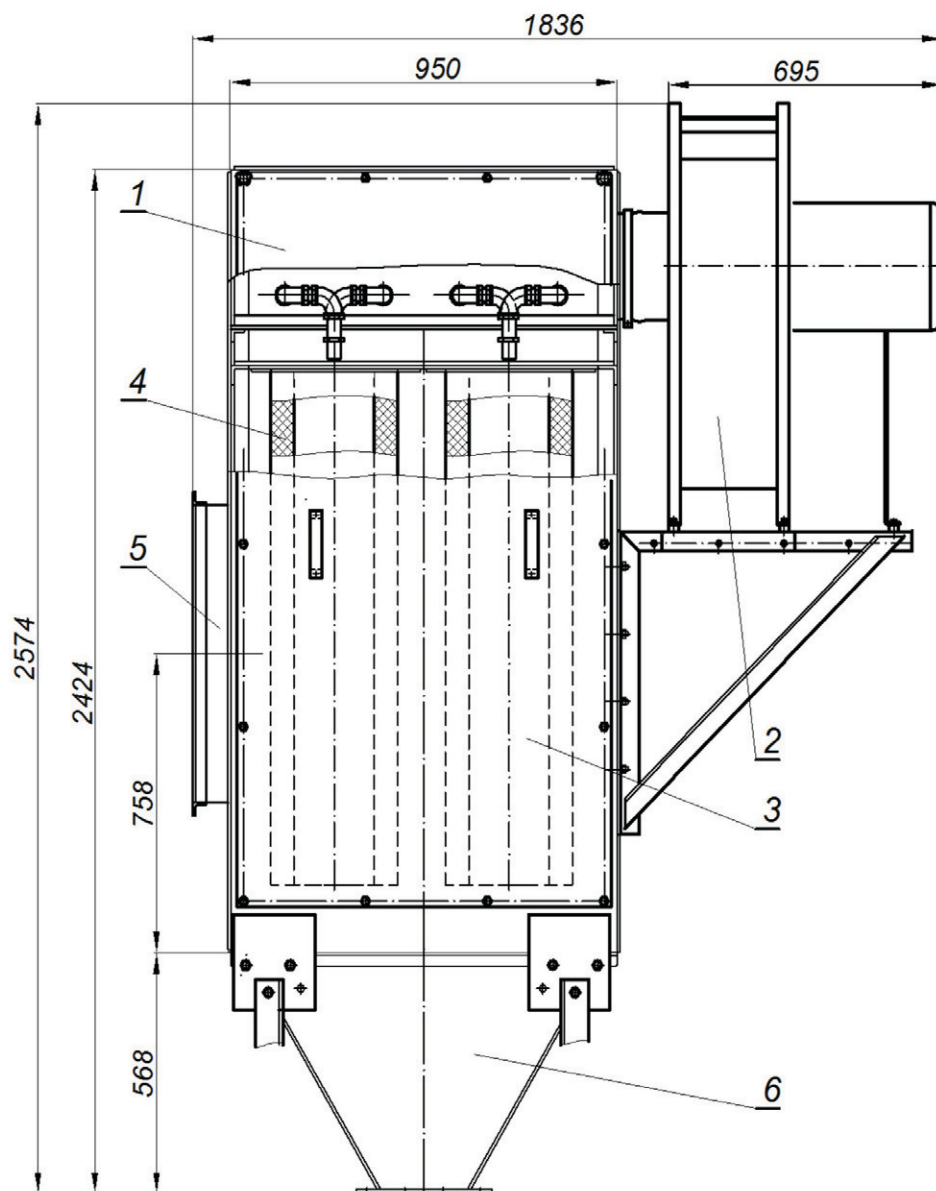
Рис. 5 Схема фильтра ФПИ-4А
