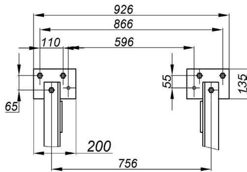
Рис. 4 Присоединительные размеры опор.
