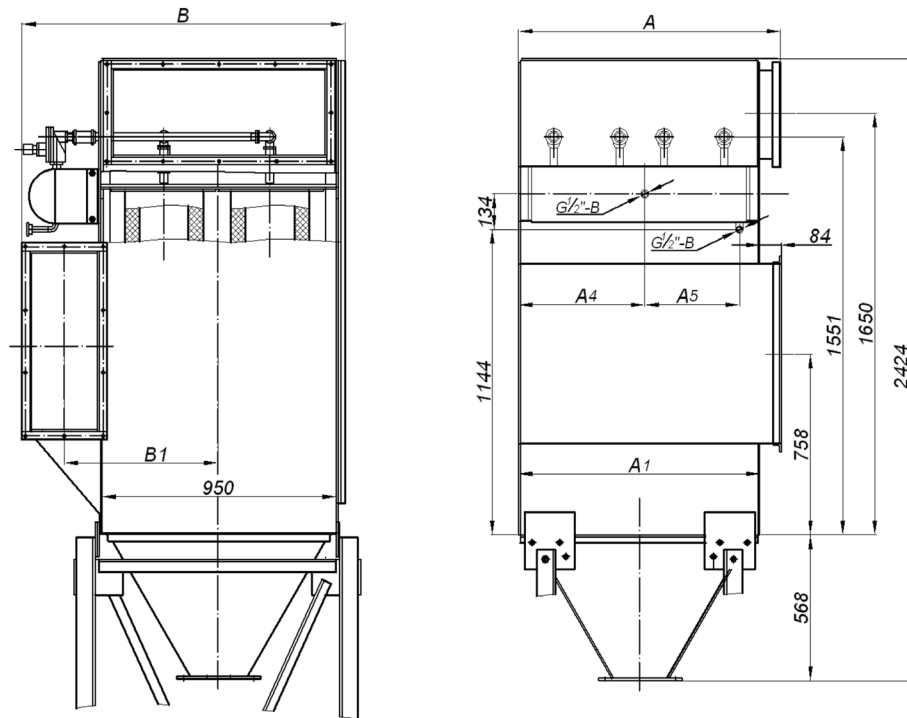
Рис. 6 Схема фильтра ФПИ-4
