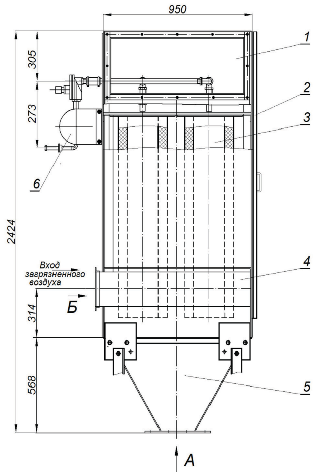
Рис. 2 Схема фильтра ФПИ-2 1 - камера чистого воздуха; 2 - дверь; 3 - фильтрующий патрон; 4 - входной патрубок; 5 - опора
