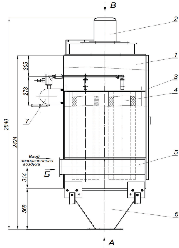
Рис. 3 Схема фильтра ФПИ-2А
