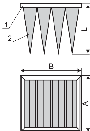
Рис.1 Схема фильтра ФЯК.
