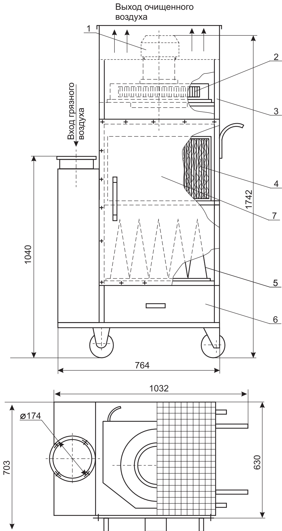
Рис. 2 Схема агрегата ПАР-М
